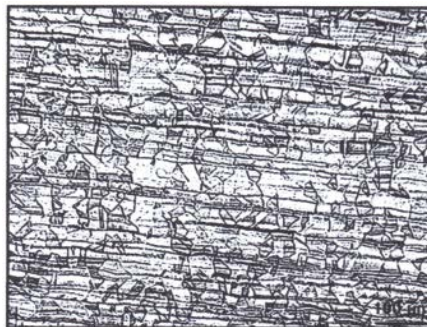
Slika 9. Struktura OM 1.4404 - TIG [7]
