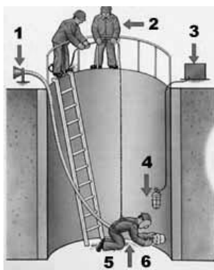
Slika 4. Zavarivanje u ograničenom prostoru (1- prijenosni ventilacijski agregat, 2 - promatrači koji nadziru, 3 - izvor napajanja, 4 - rasvjetna lampa, 5 - spasilačko uže, 6 - zavarivač) [17]
